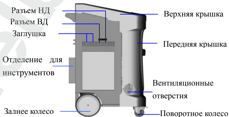
Вид слева
